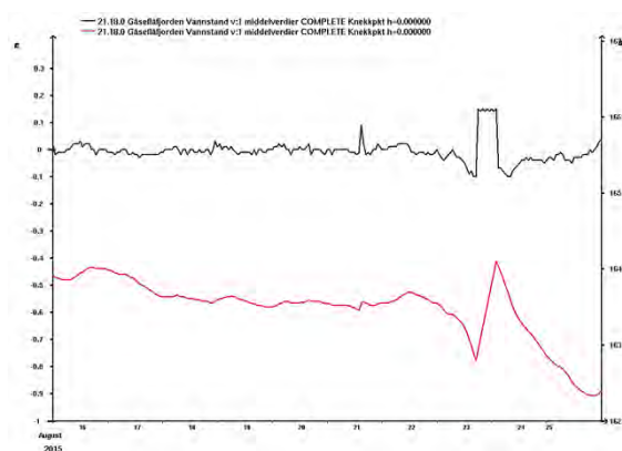
Figur 7. Observert vannstand Gåseflåfjorden (timesverdier) i august 2015 (rød strek) og endring fra time til time (svart strek).
