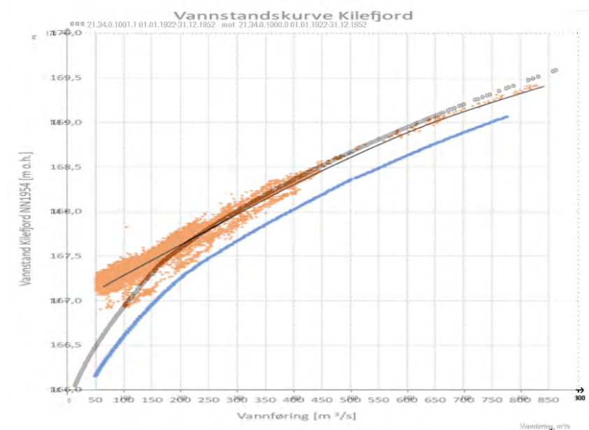
Figur 1. Kopi av figur 15 fra SINTEFs rapport, hvor blå «punkter» skal vise kapasiteten i Soga før bygging av Gåseflådamme og oransje punkter dagens kapasitet. I tillegg er det lagt inn vannstand/ vannføring fra NVEs database Hydra II for Kilefjord målestasjon for årene 1922-1952 (før utbygging), som svarte punkter. De svarte punktene ligger drøyt 30 cm høyere enn de blå «punktene» fra SINTEF.
